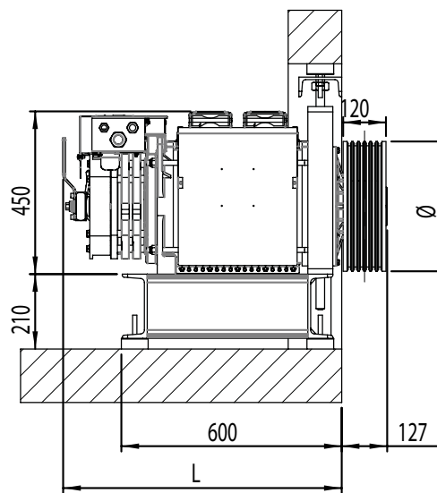
SEZIONE A-A
